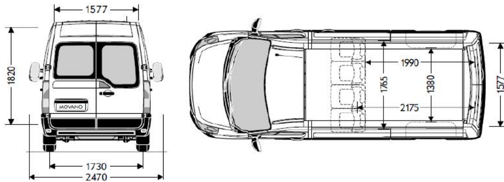
Furgone Doppia Cabina L2H2 – T. Anteriore
